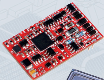
56630 PSD XP Sound BR 62 PluX22 & Lautsprecher
