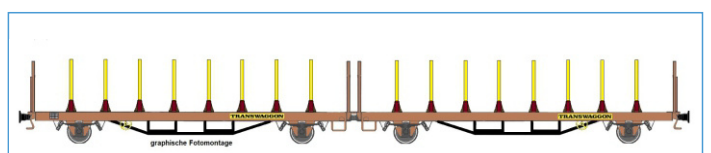
4achsige Flachwagen-Doppelunit Bauart Laas 1 der Fa. Transwaggon eingestellt bei der DB AG (Ep.V/VI) rotbraun einfarbig, unbel., ExTe-Rungen, gelb
