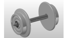
NZ 33273 Scheibenrad 10mm, schmal, AZ 13,2mm spitzengel., eins. isoliert
