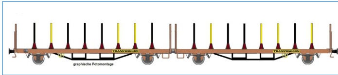
4achsige Flachwagen-Doppel­einheit Bauart Laas 1 der Fa. Transwaggon eingestellt bei der DB AG (Ep.V/VI) rotbraun einfarbig, unbel., ExTe- Rungen, gelb-schwarz
