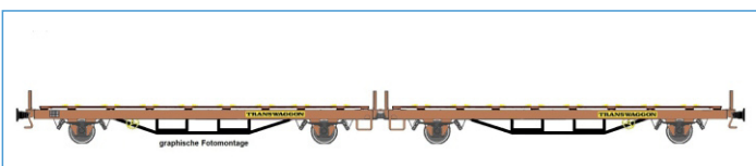
4achsige Flachwagen-Doppelunit Bauart Laas 1 der Fa. Transwaggon eingestellt bei der DB AG (Epoche V/VI) rotbraun einfarbig, unbeladen, mit Halter für Radfahrzeuge
