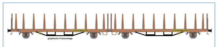
4achsige Flachwagen-Doppelunit Bauart Laas 1 der Fa. Transwaggon eingestellt bei der DB AG (Epoche V/VI) rotbraun einfarbig, unbeladen
