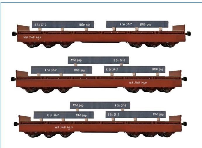
6-achsiges Schwerlastwagen-Set Bauart Samms 4860 der DR (Epoche IV) Transportzug Stahlwerk Brandenburg 3 Wagen beladen mit Stahlbrammen Wagen 1: braun einfarbig Wagen 2: braun-braun-schwarz Wagen 3: braun-schwarz-schwarz NW 22406 DC 2L H0 169,90 €
