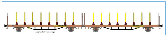
4achsige Flachwagen-Doppel Einheit Bauart Laas 1 der Fa. Transwaggon eingestellt bei der DB AG (Epoche V/VI) rotbraun einfarbig, unbeladen ExTe-Rungen, gelb NW 52207 DC 2L TT 1. B.Nr. 119,90 €
